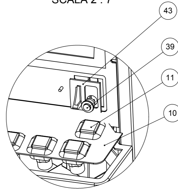
DETTAGLIO A SCALA 2 : 7
